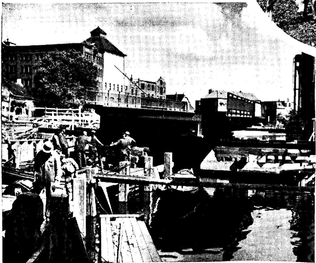
DE DOORVAARTOPENING DER BONTEBRUG is tijdelijk voor de scheepvaart ge- stremd tijdens het plaatsen van de nieuwe brug op haar onderbouw.
