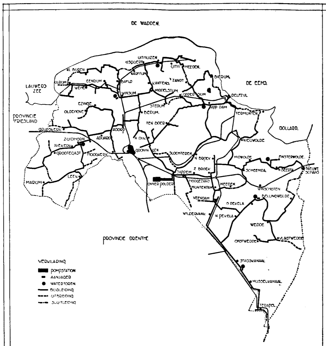
Overzicht van de buisleiding der Provinciale Groningsche Waterleiding.
