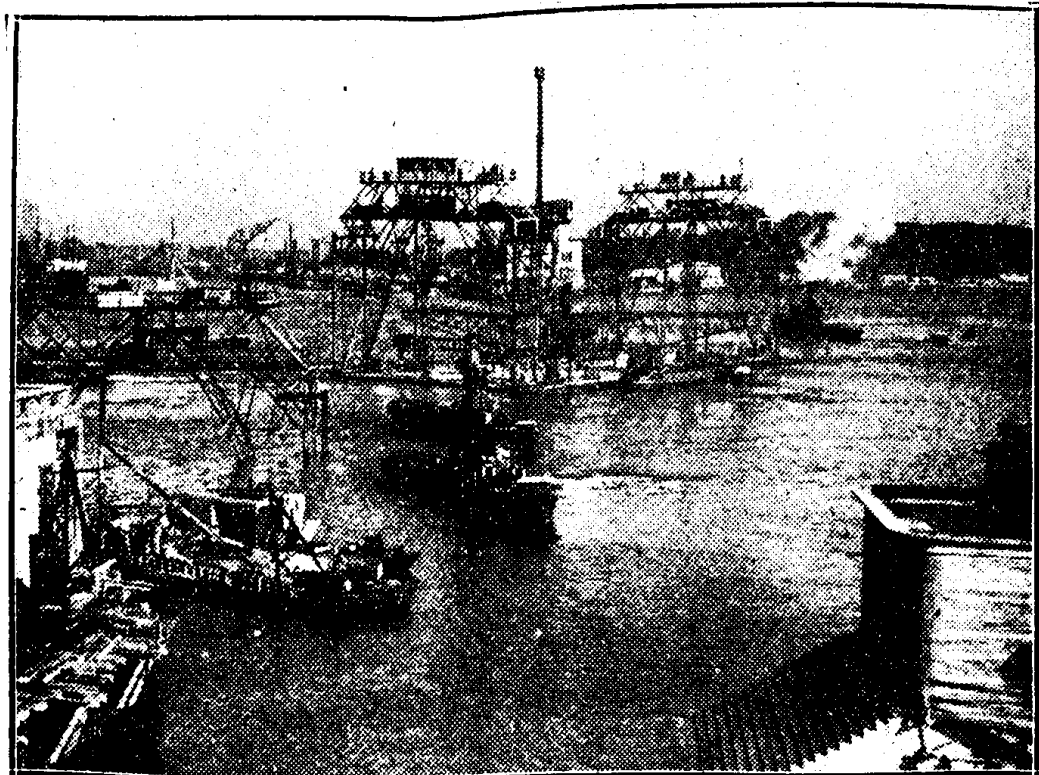
De Maastunnelbouw is weer een belangrijke etappe gevorderd. Het achtste tunnelstuk van de Waalhaven is versleept naar de plaats waar het tot zinken zal worden gebracht, n.l. tegen het negende tunnellement, dat reeds op de definitieve plaats tegen het ventilatiegebouw op den linker Maasoever ligt. Overzicht van het transport. (Polygoon).
