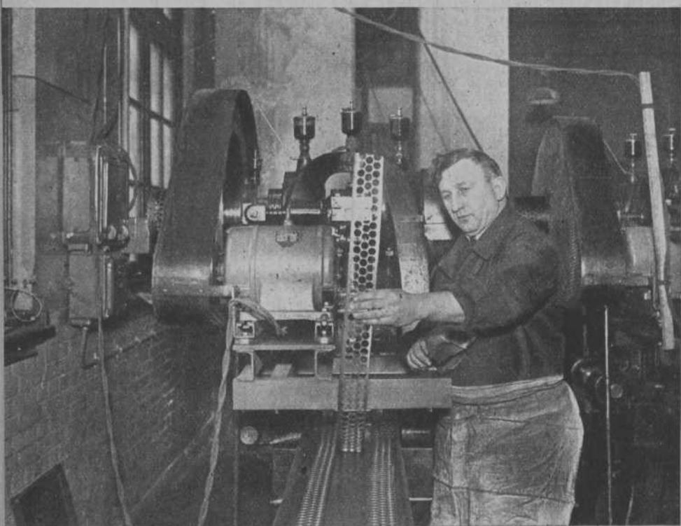
Hier worden de centen in hun „oervorm” gemaakt: de ponsmachine slaat uit lange koperen platen tal van metaalcirkeltjes.
