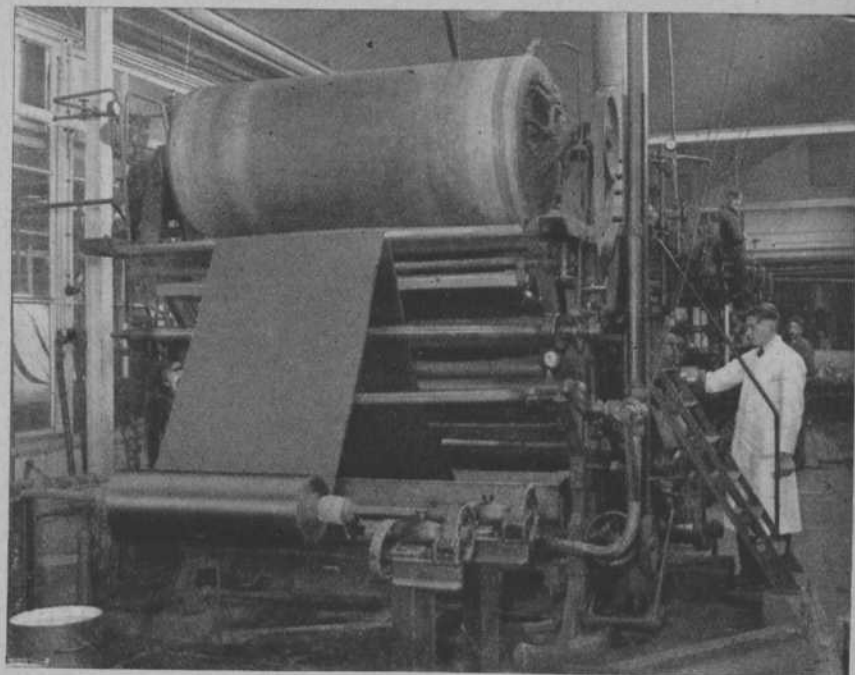
Een moderne spanmachine.
