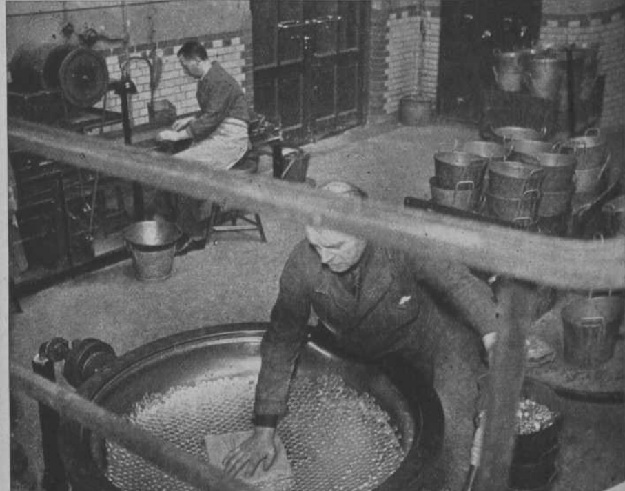
In een stoompan met dubbelwand heeft het drogen plaats. De „zilverpracht” wordt schoon gepoetst.
