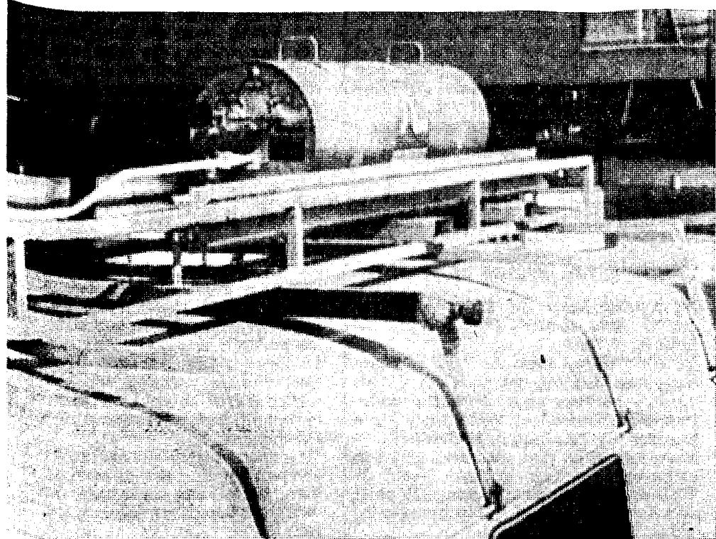
Een tank voor vloeibaar aardgas met een inhoud van 45 liter, bevestigd op het dak van een van de proefauto's.
